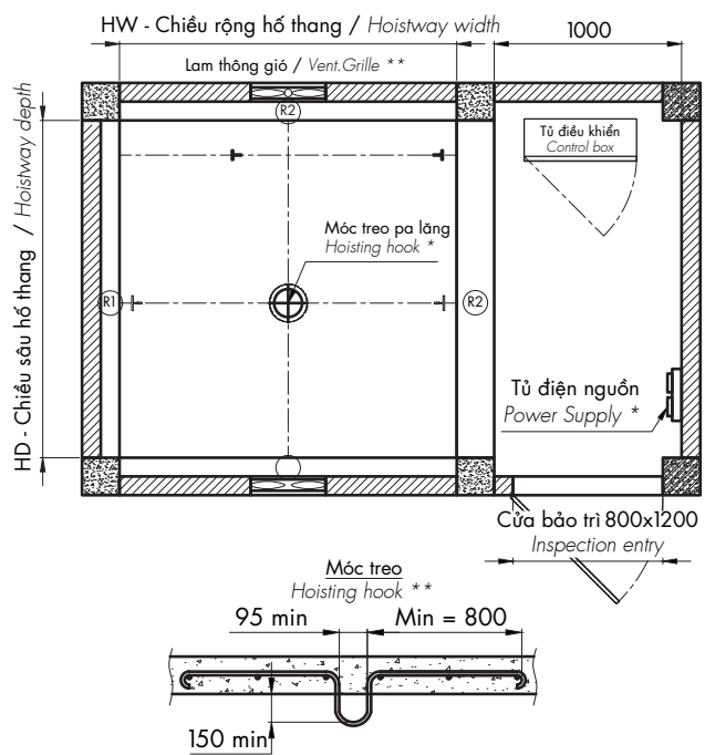
Mặt bằng phòng máy Machine room plan
