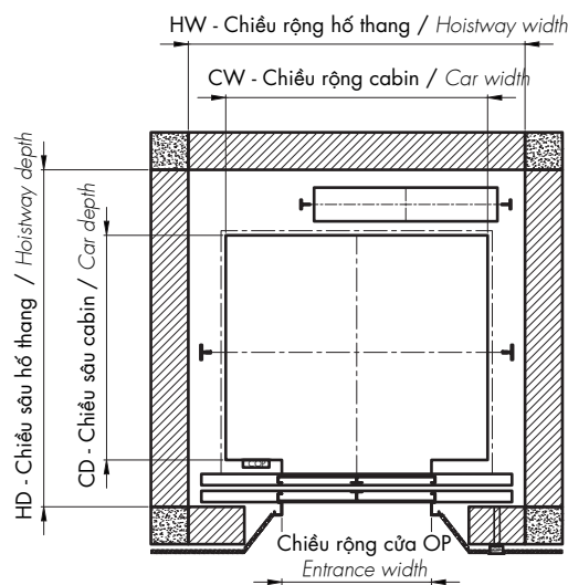
Mặt bằng điển hình Typical plan
